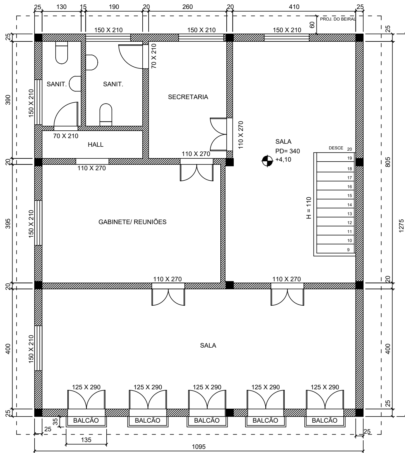
PLANTA 2º PAVTO. ESC.: 1:75
