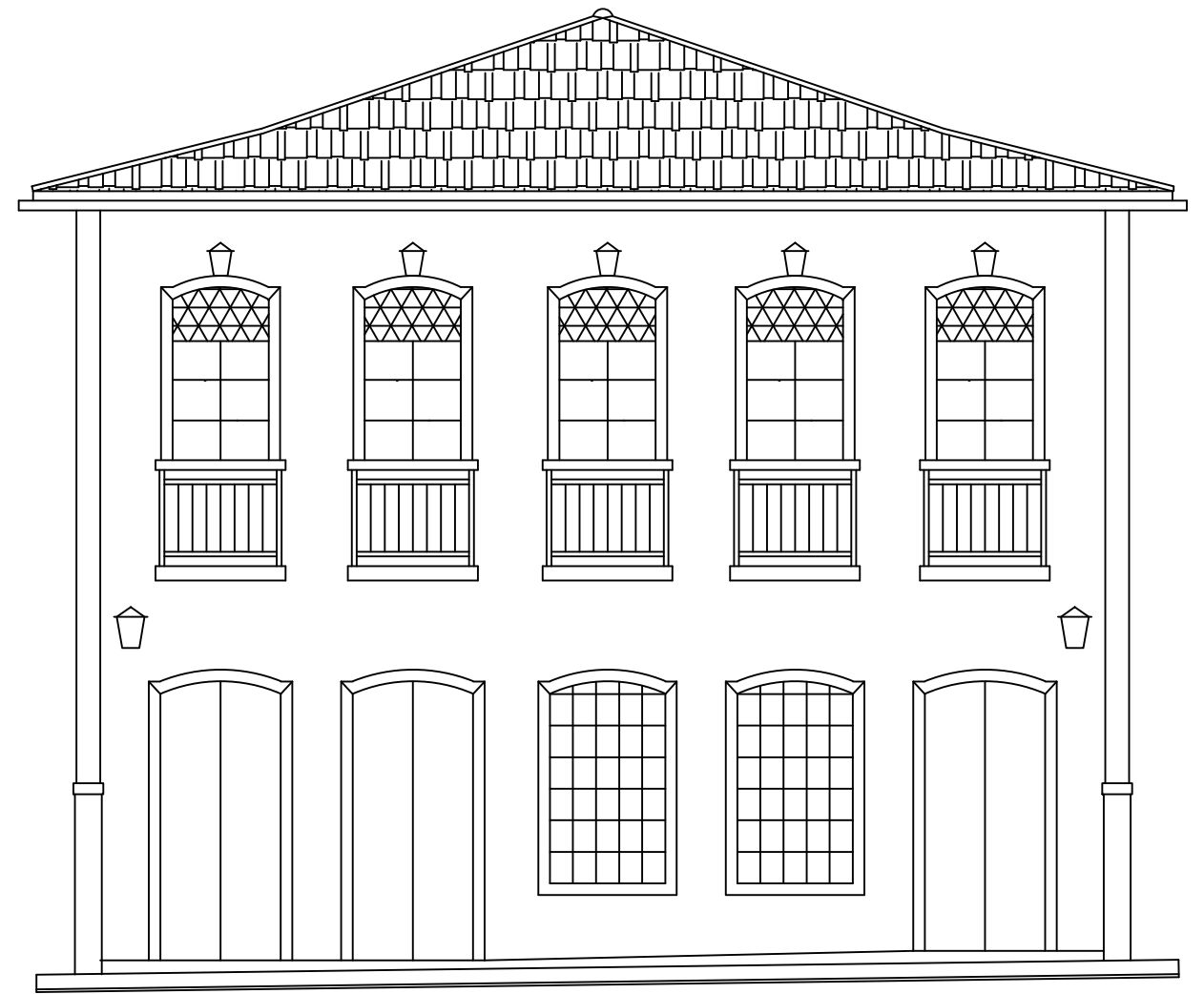
FACHADA ESC.: 1:75
