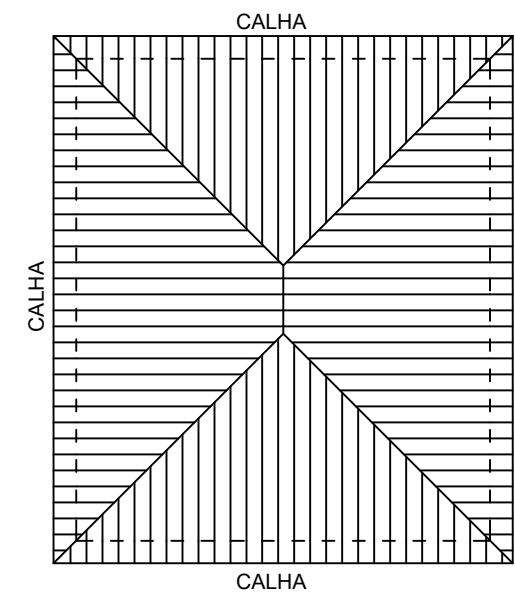
DIAGRAMA DE COBERTURA i= 30% ESC.: 1:200
